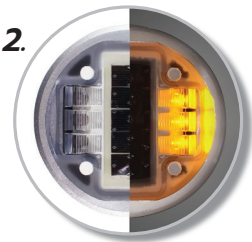
2. ด้านในมีไฟ LED ความสว่างสูง 6 ดวง
