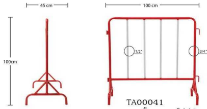
TA00041 แผงกั้นจราจร ไม่มีล้อ 1 เมตร
